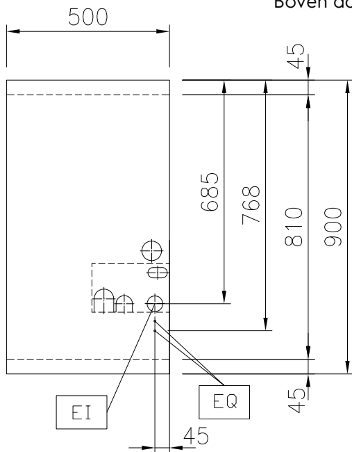
Boven aanzicht
